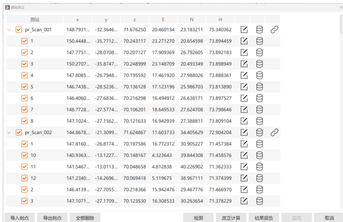
图 3-67 测站改正
